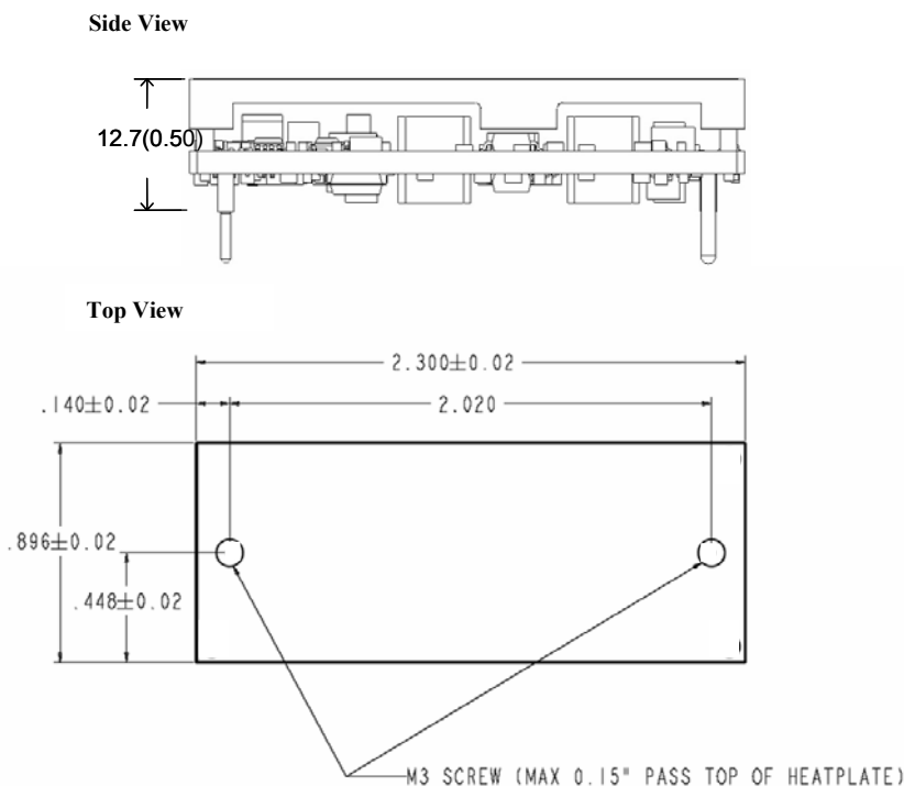
Fig. 17. Open Frame Converter
